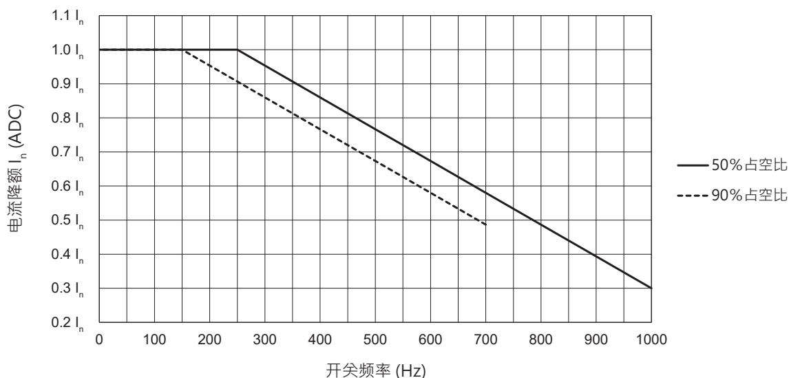
Fig. 6 电流降额vs开关频率 5
