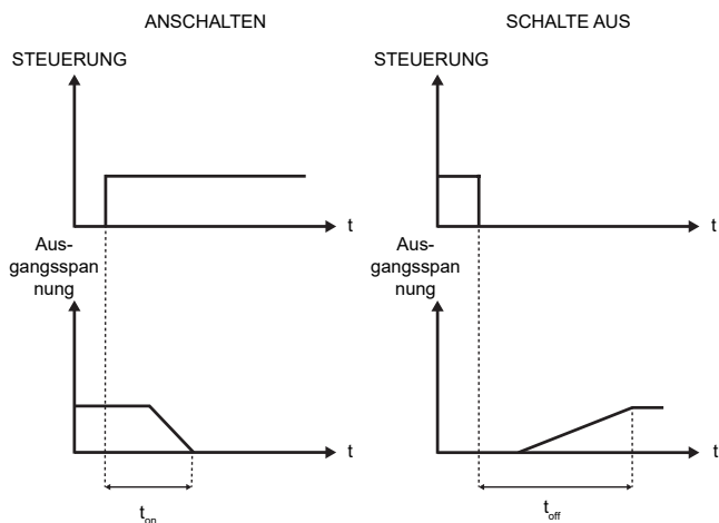
Fig. 2 Reaktionszeitmerkmale
