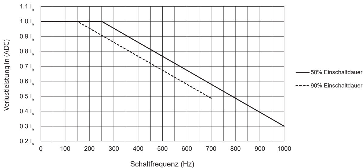
Fig. 6 Strom-Derating und Schaltfrequenz 5
