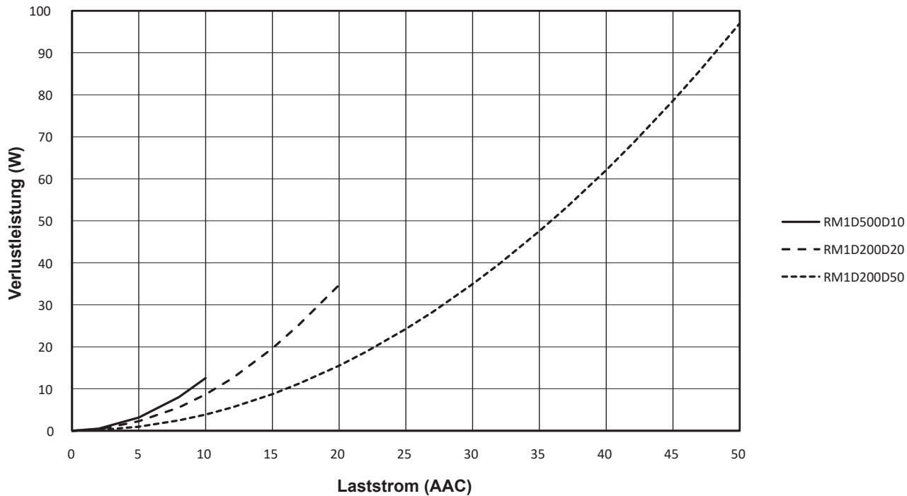
Fig. 9 Verlustleistungskurve
