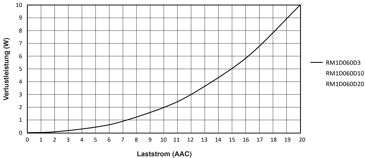
Fig. 7 Verlustleistungskurve
