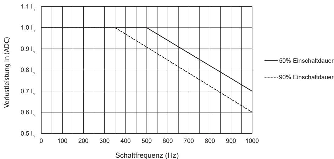
Fig. 4 Strom-Derating und Schaltfrequenz
