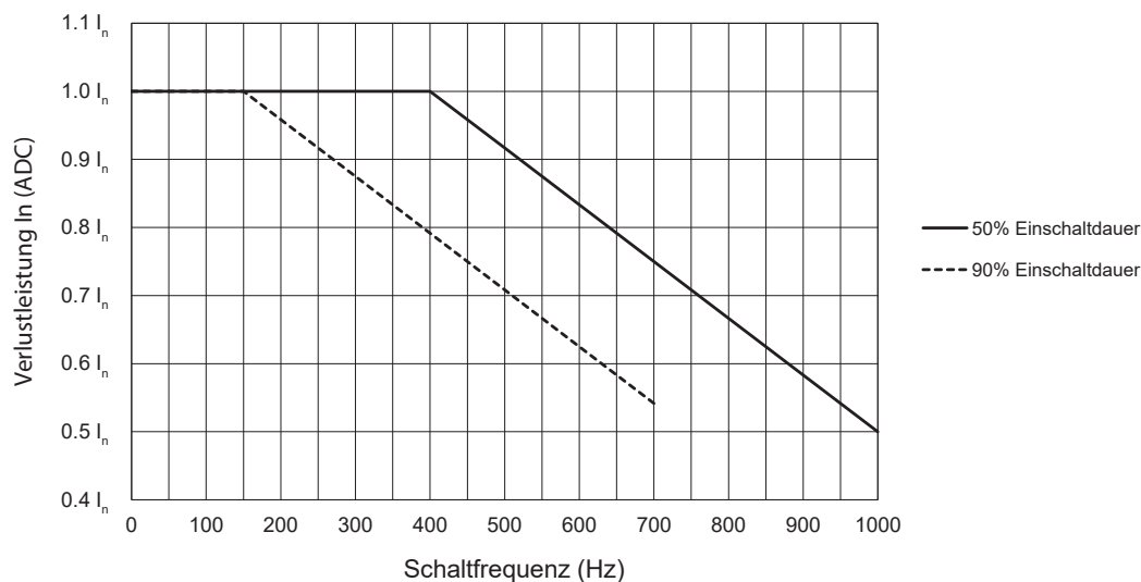
Fig. 5 Strom-Derating und Schaltfrequenz 4
