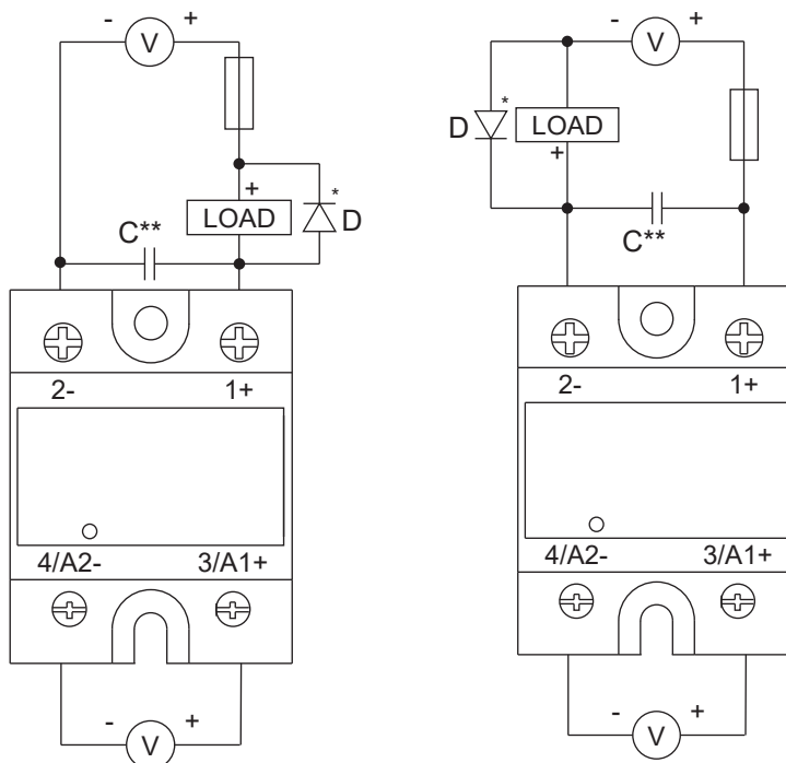
Fig. 10 RM1D-Anschlussschaltpläne
