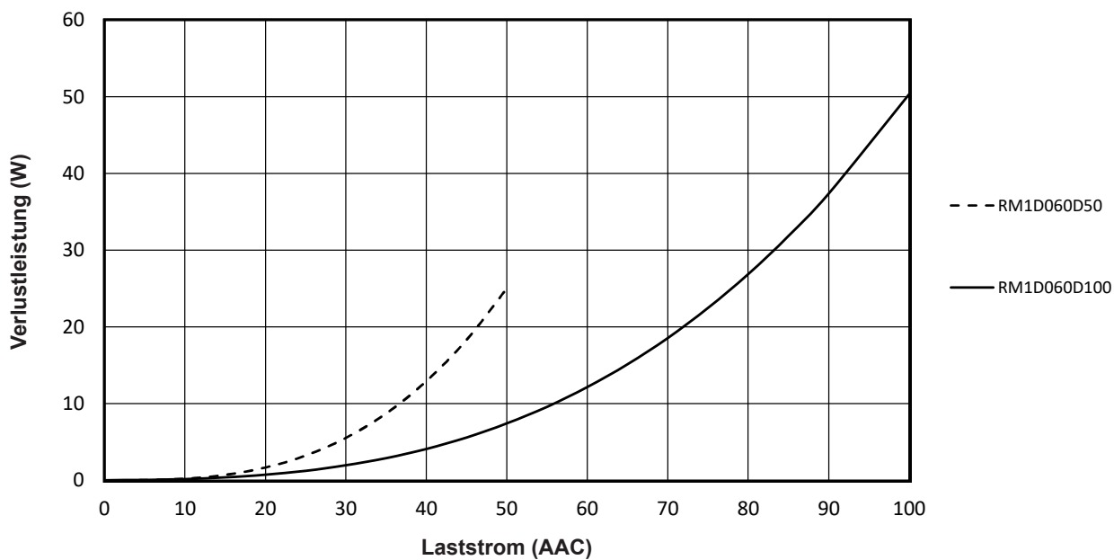
Fig. 8 Verlustleistungskurve
